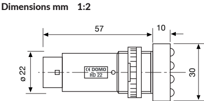
Dimensions mm 1:2
