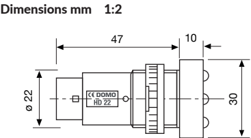
Dimensions mm 1:2
